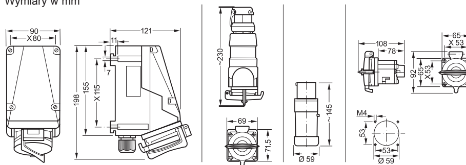
Gniazdo natynkowe
